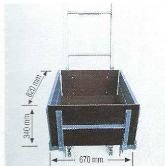
Transportbühne mit abklappbarem Seitenschutz und einstellbarer Bühneneigung.
