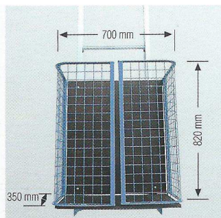
Universalpritsche mit klappbarem Schutzgitter – das Vielzwecktransportmittel!
